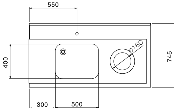
Boven aanzicht
